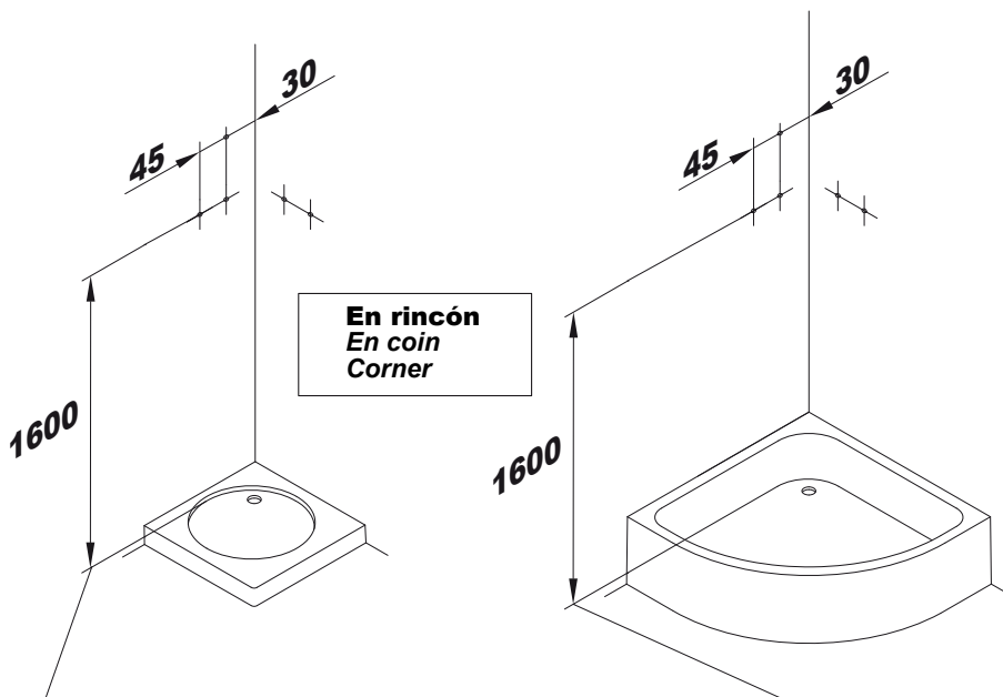
Cotas tomadas desde el fondo del plato o bañera
