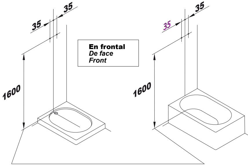
Cotas tomadas desde el fondo del plato o bañera
